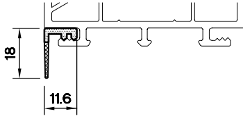
KAPAMA PR. (18) 1399.372
