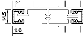
BAĞ PR. (14) 1399.212
