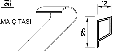
KENAR PR.
