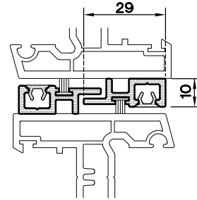
ARA SIZDIRMAZLIK PR. 13S1.102
