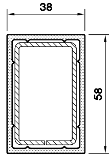
PVC KUTU PR. ( 40 X 60 )
