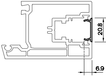
KANAT KAPAMA PR. 13S1.101
