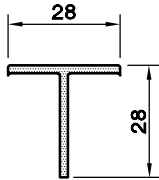
T - PR. ( 28 x 28 )
