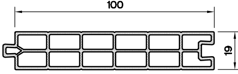
LAMBRİ PR. ( 19 x 100 )
