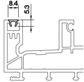
KANAL KAPAMA PR. 13S2.103
