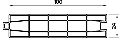
LAMBRİ PR. ( 24 x 100 )
