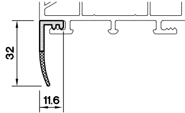
GENİŞ KAPAMA PR. (32) 1399.373
