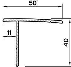
T - PR. ( 40 X 50 )
