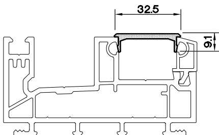
DOLGU PR. 13S2.101
