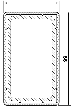
PVC KUTU PR. ( 60 X 100 )
