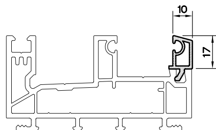
ÇİFTCAM ÇİTASI 12S3.110
