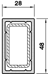
PVC KUTU PR. ( 30 X 50 )
