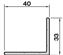
L - PR. ( 33 X 40 )
