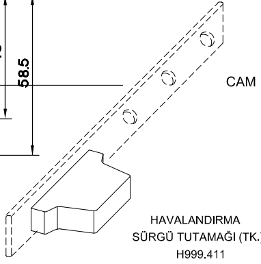
HAVALANDIRMA PR. SETİ
