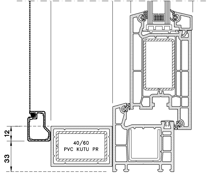
KESİT
