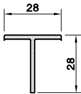
T - PR. ( 28 x 28 ) 1399.351
