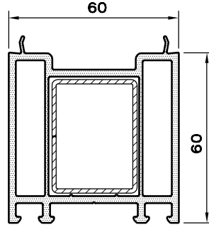
KASA UZATMA PR. (60) 1399.263
