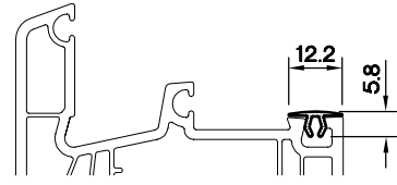
KANAL KAPAMA PR. 1399.101
