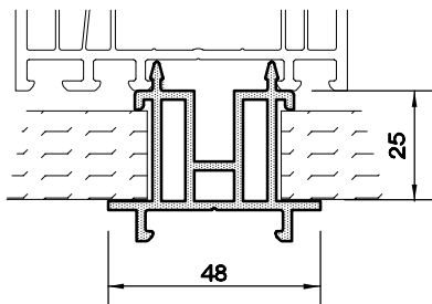
KASA TABAN PR. 1399.251
