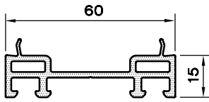
KASA UZATMA PR. (15) 1399.261
