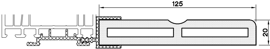
AL. PARAPET ADAPTÖR PR. 6599.201
