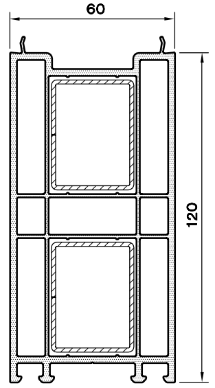
KASA UZATMA PR. (120) 1399.264
