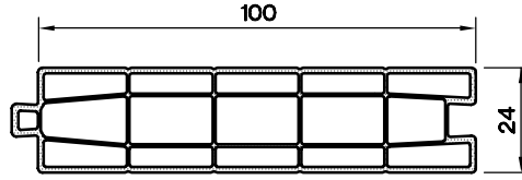
LAMBRİ PR. ( 24 x 100 ) 1399.117
