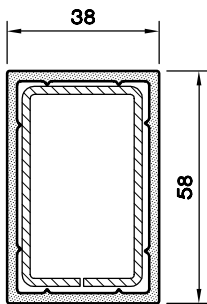
PVC KUTU PR. ( 40 X 60 ) 132.925
