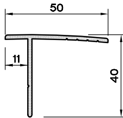
T - PR. ( 40 X 50 ) 1399.353
