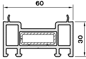
KASA UZATMA PR. (30) 1399.262
