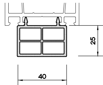
TIRNAKSIZ KASA TABAN PR. 1399.252
