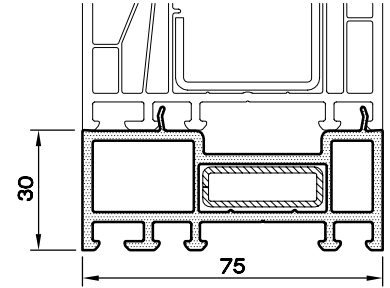
KASA UZATMA PR. (30) 1375.262
