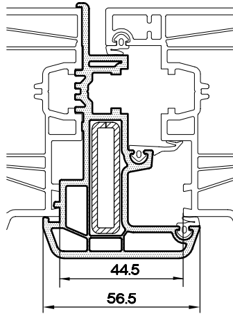
ÇİFT KANAT BİNİ PR. 1375.111
