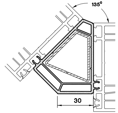
135° KÖŞE DÖNÜŞ PR. 1399.233
