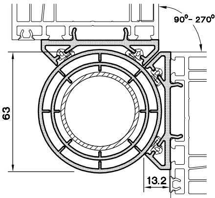
KÖŞE DÖNÜŞ PR. ( 60 ) 1399.230
