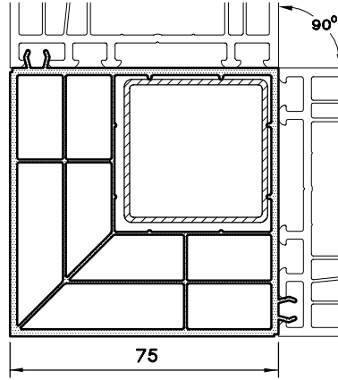
90° KÖŞE DÖNÜŞ PR. 1375.231
