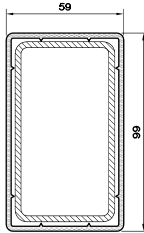
PVC KUTU PR. ( 60 X 100 ) 1399.223
