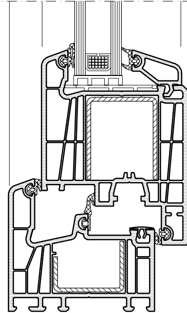
KESİT
