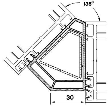
135° KÖŞE DÖNÜŞ PR.
