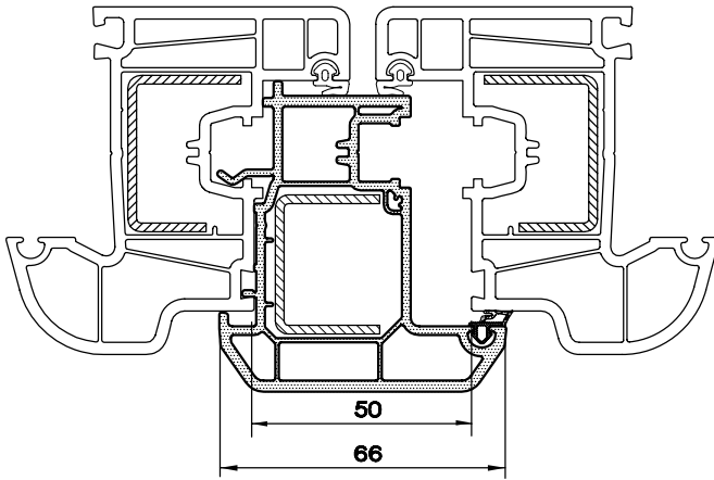
ÇİFT KANAT BİNİ PR. 1370.111
