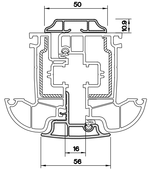
ÇİFT KANAT İÇ KAPAMA PR. 1371.113
