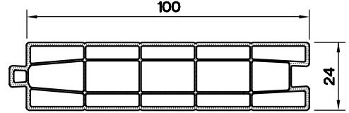
LAMBRI-24 x 100 PR. 1399.117
