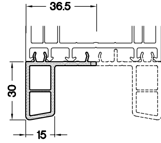
PARAPET KAPAMA PR. 1399.378
