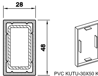
PVC KUTU-30X50 KAPAK PARC. E399.335
