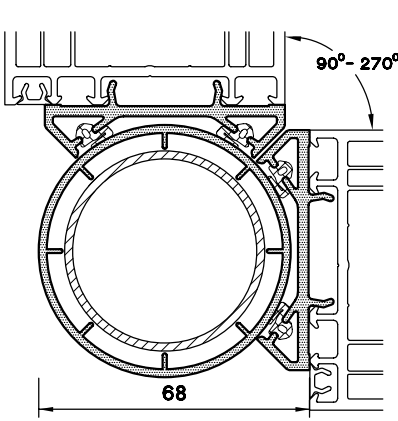
KÖŞE DÖNÜŞ-60 PR.
