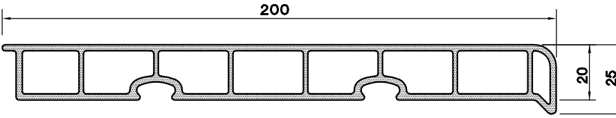
PARAPET-200 x 25 PR. 1399.337
