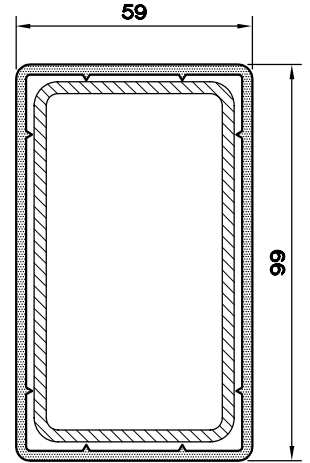
PVC KUTU- 60 X 100 PR.
