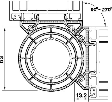
KÖŞE DÖNÜŞ-60 PR.
