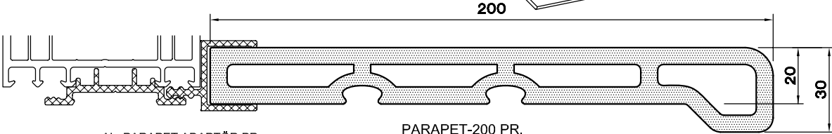
AL. PARAPET ADAPTÖR PR. 6599.201 PARAPET-200 PR. 1399.336
