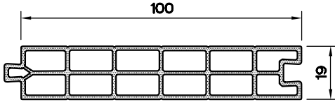
LAMBRI-19 x 100 PR. 1399.115
