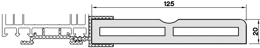
AL. PARAPET ADAPTÖR PR. 6599.201 PARAPET-125 PR. 1399.335
