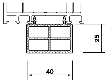
KASA TABAN PR. 1399.252
