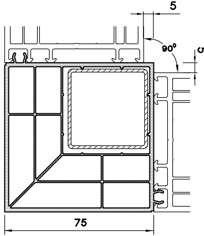
90° KÖŞE DÖNÜŞ PR.
