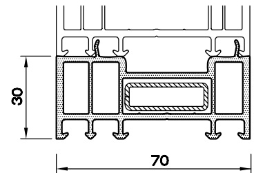
KASA UZATMA-30 PR. 1370.130 KUTU PR. (10 X 30 X 1.5mm) 5160.321
