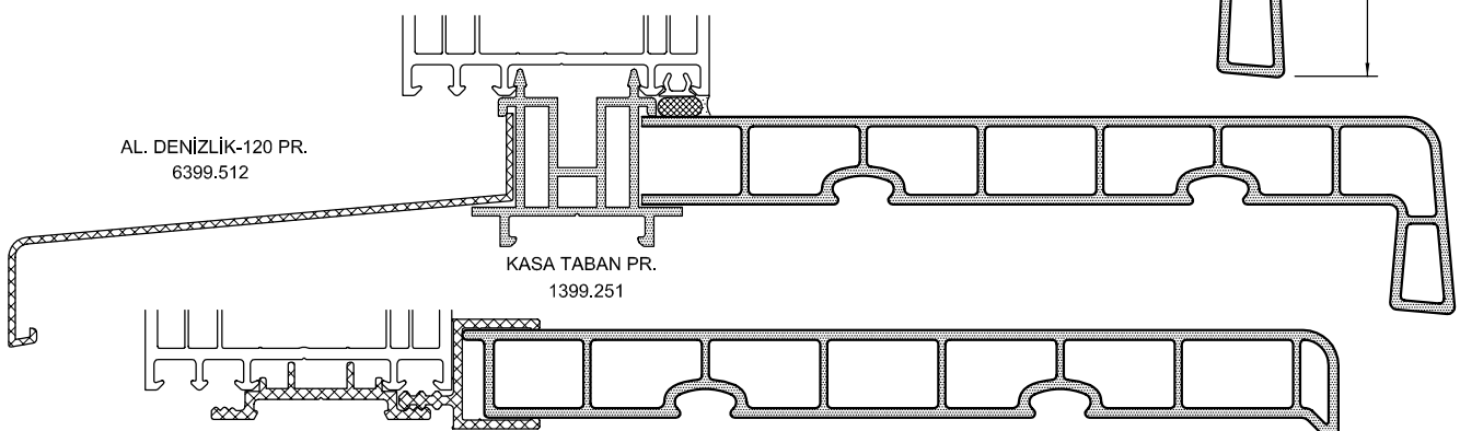
PARAPET-300 x 70 PR. 1399.339
