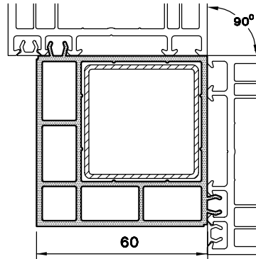
90° KÖŞE DÖNÜŞ PR.
