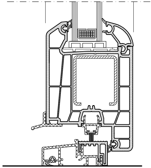
KESİT
