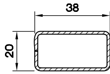
KUTU PR. (20X38-2.0) 5399.212
