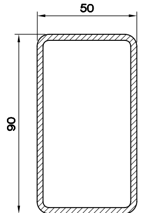
KUTU PR. (50X90-2.0) 5399.232
