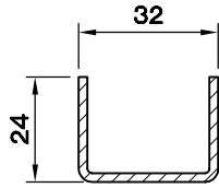
U DESTEK SACI 32X24 (1.5) 5161.911
