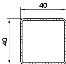
KUTU PR. (40X40-1.5) 5399.411
