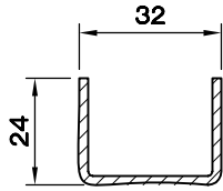
U DESTEK SACI 32X24 (2.0) 5161.912
