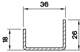
U DESTEK SACI 36X18X26 (2.0) 5175.912
