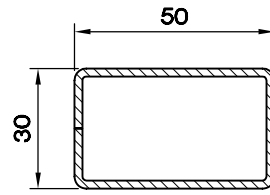
KUTU PR. (30X50-2.0) 5399.222
