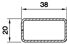
KUTU PR. (20X38-1.5) 5399.211
