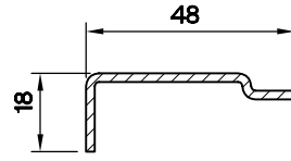
BİNLİ KANAT-49/3 DESTEK SACI (1.5) 5170.211
