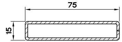
KUTU PR. (15X75-2.0) 5399.112
