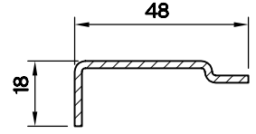
BİNLİ KANAT-49/3 DESTEK SACI (2.0) 5170.212
