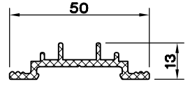
AL. ADAPTÖR -50 PR. 6599.301
