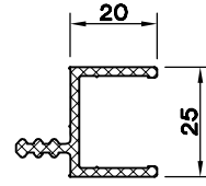
AL. PARAPET ADAPTÖR PR. 6599.201
