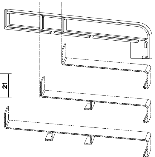
AL. DENİZLİK KAPAK PARÇA TK. E399.327
