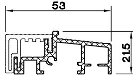
AL. EŞİK PR. 6353.101
