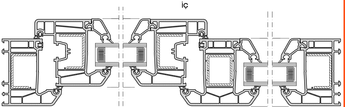
KESİT
