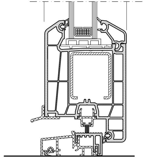
KESİT
