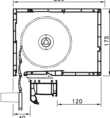
Y. PANJUR KUTU PR. SETİ (210) 210
