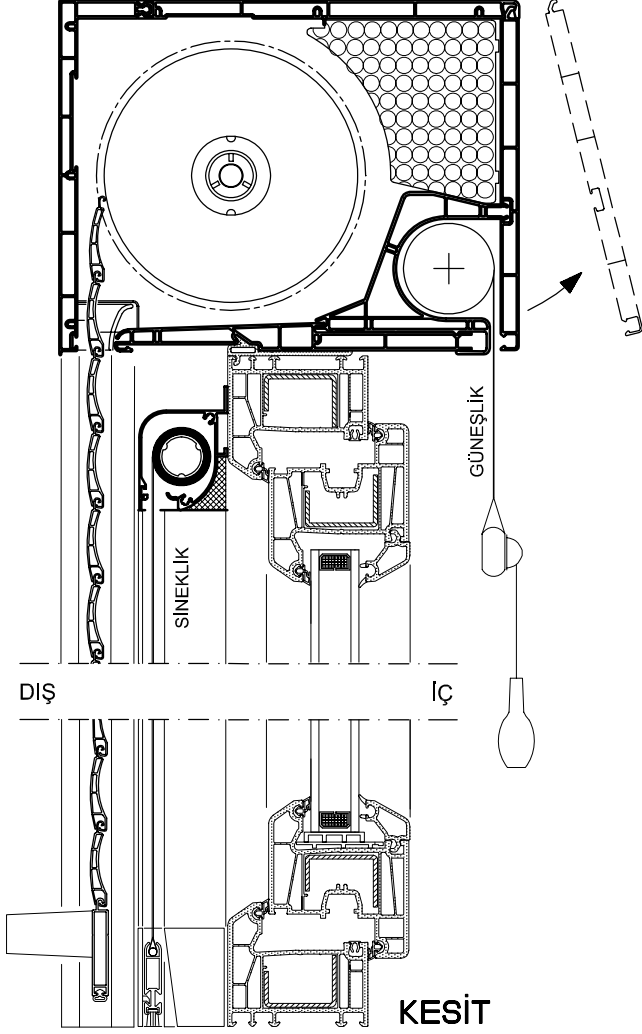
SABİT PANJUR (Güneşlik ve Sineklikli) PANJUR KUTU PR. SETİ (175)
