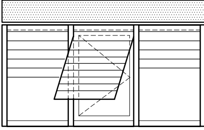
PANJUR KUTU PR. SETİ (210) 260
