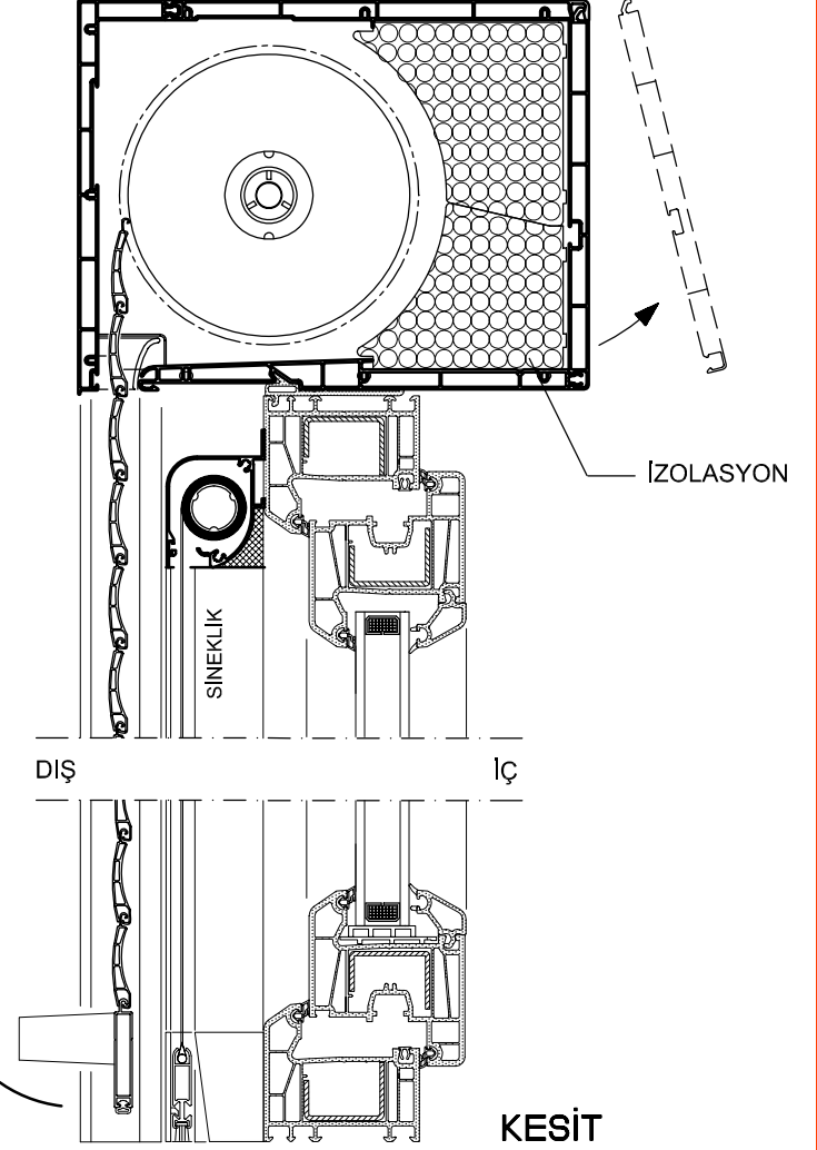
AÇILIR PANJUR (Sineklikli) PANJUR KUTU PR. SETİ (175)
