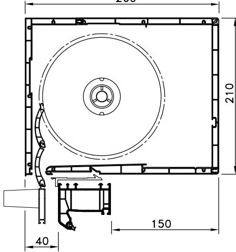
PANJUR KUTU PR. SETİ (175) 230
