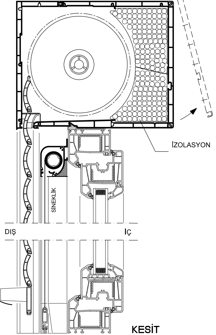
AÇILIR PANJUR (Sineklik) PANJUR KUTU PR. SETİ (210)
