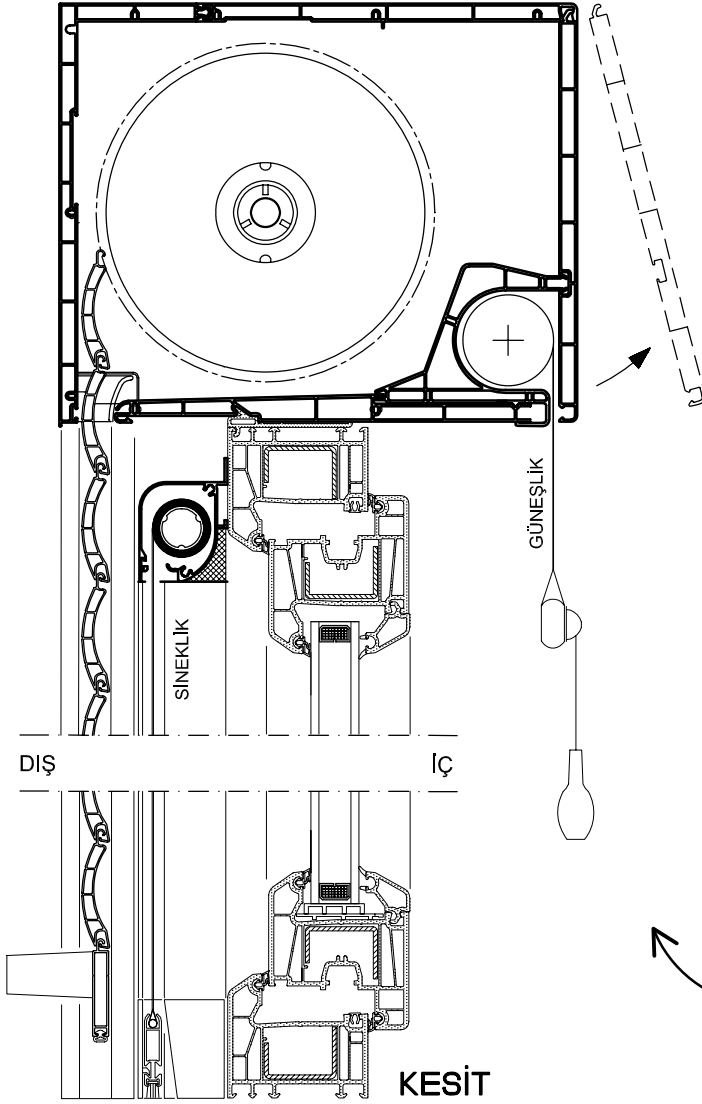
SABİT PANJUR (Güneşlik ve Sineklik) PANJUR KUTU PR. SETİ (210)
