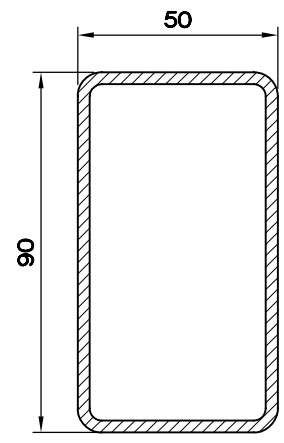
KUTU PR.(50X90-2.0) 5399.232
