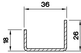
U DESTEK SAÇI 36X18X26 (2.0) 5175.912
