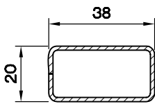
KUTU PR.(20X38-1.5) 5399.211
