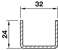
U DESTEK SAÇI 32X24 (1.5) 5161.911
