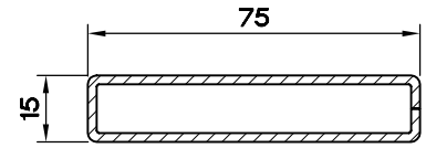
KUTU PR. (15X75-2.0) 5399.112
