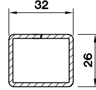
ORTAKAYIT-81/3 DESTEKSACI (2.0) 5153.322
