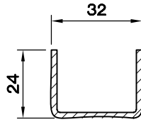
U DESTEK SAÇI 32X24 (2.0) 5161.912
