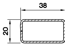
KUTU PR.(20X38-2.0) 5399.212
