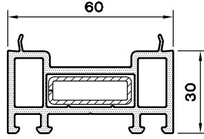
KASA UZATMA PR. (30) 1399.262
