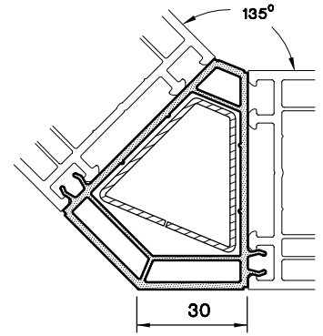
135° KÖŞE DÖNÜŞ PR. 1399.233
