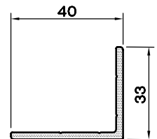
L - PR. ( 33 X 40 ) 1399.363
