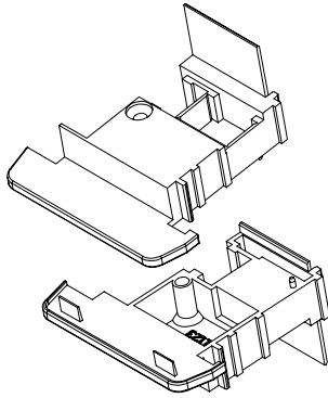
ÇİFT KANAT BİNİ PR. (13) UÇ KAPAMA PARÇASI E360.123
