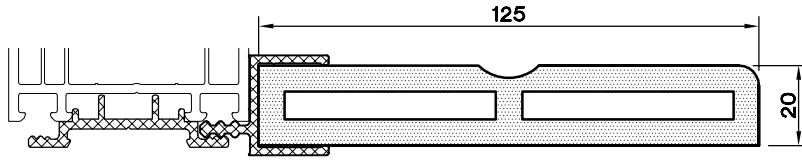
AL. PARAPET ADAPTÖR PR. 6599.201
