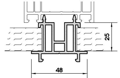
KASA TABAN PR. 1399.251
