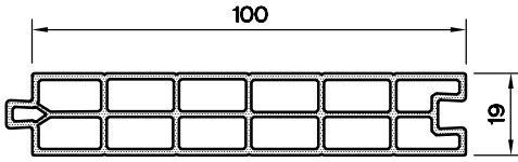
LAMBRİ PR. ( 19 x 100 ) 1399.115
