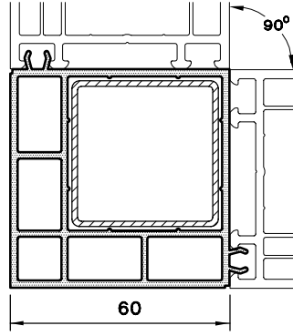
90° KÖŞE DÖNÜŞ PR. 1399.231
