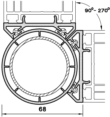
KÖŞE DÖNÜŞ PR. ( 60 ) 1399.230
