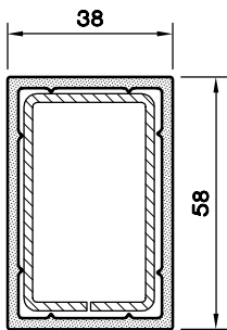
PVC KUTU PR. ( 40 X 60 ) 1399.222
