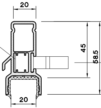
HAVALANDIRMA PR. SETİ H999.420
