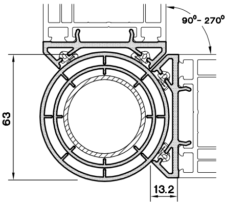
KÖŞE DÖNÜŞ PR. ( 60 ) 1399.230
