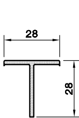
T - PR. ( 28 x 28 ) 1399.351
