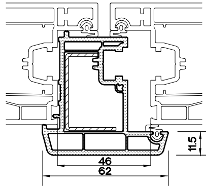
ÇİFT KANAT BİNİ PR. (13) 1361.101
