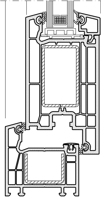
KESİT
