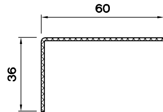
GENEL DESTEK SACI 36x60-1.5 59213010000000000
